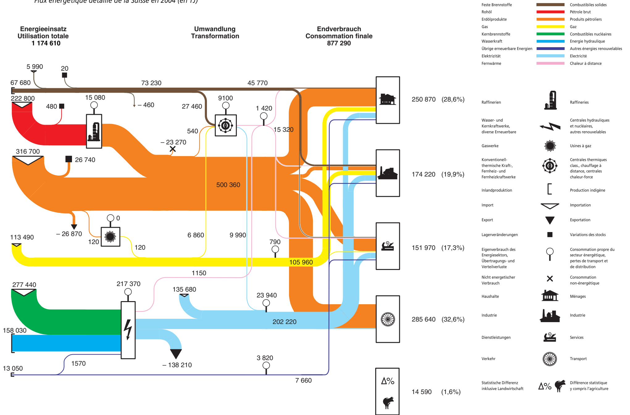
Fig. 5 Detailliertes Energieflussdiagramm der Schweiz 2004 (in TJ) Flux énergétique détaillé de la Suisse en 2004 (en TJ)
