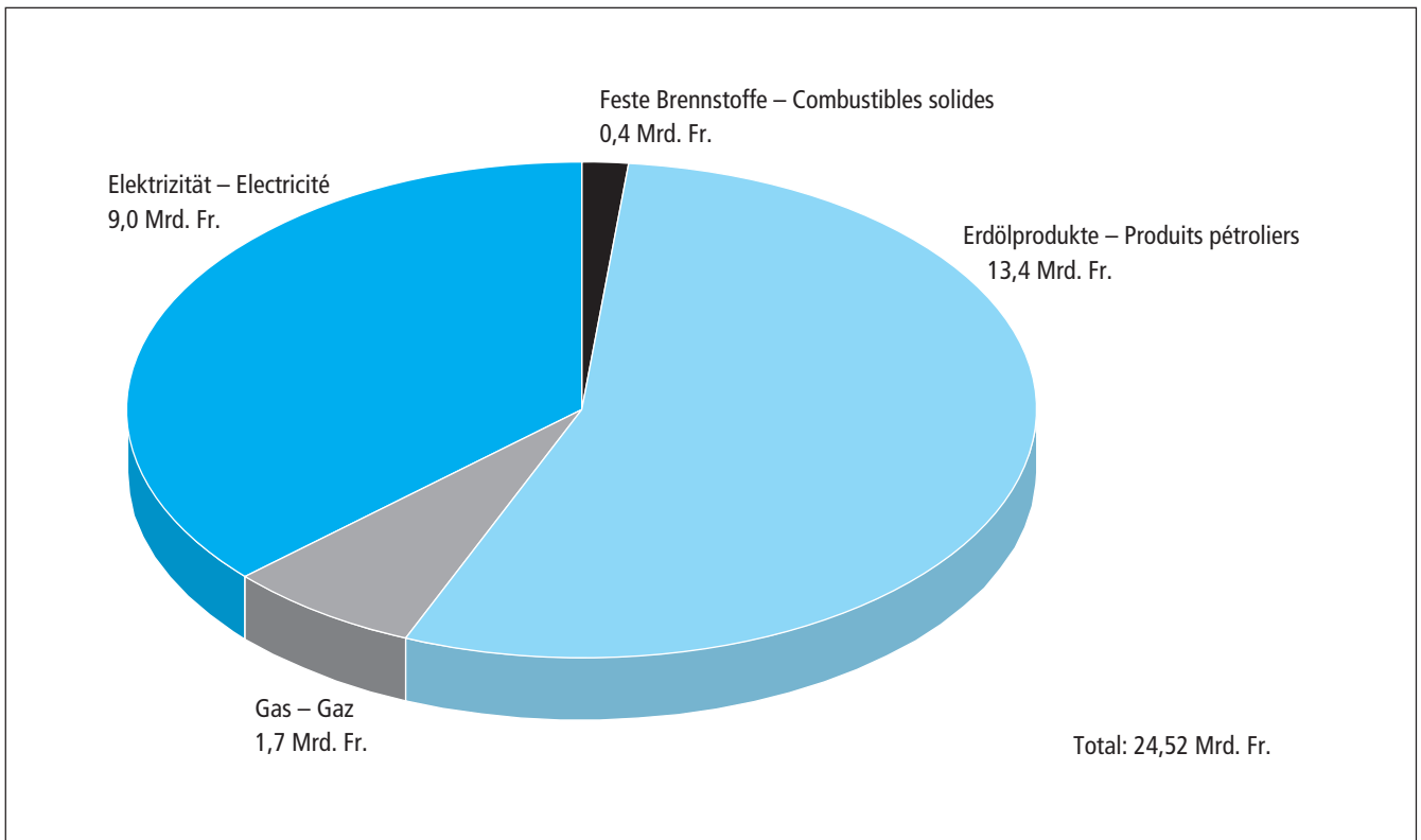
Fig. 13 Endverbraucher-Ausgaben für Energie 2004 Dépenses des consommateurs finaux d'énergie 2004
