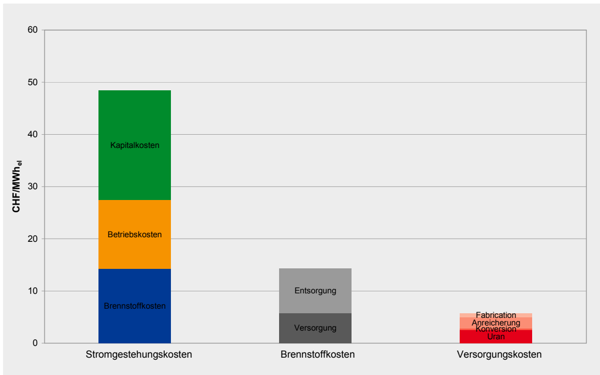
Abbildung 1: Zusammenstellung der Stromgestehungskosten von neuen Kernkraftwerken
